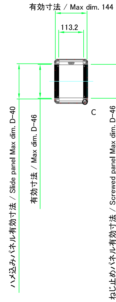
ナットレール / Nut rail
